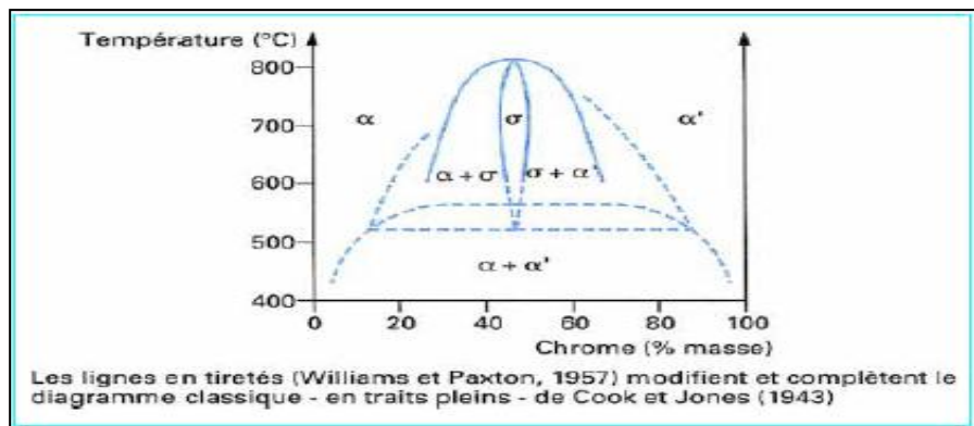
Figure 1.5. – Diagramme d'équilibre Fe – Cr au-dessous de 800 °C : domaine d'existence des phases \alpha \alpha' et \sigma [21]
