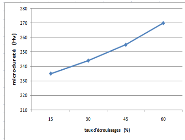
Figure 3.14. Déformation à froid après un maintien de 15 min à 900°C suivi d'un refroidissement à l'air.
