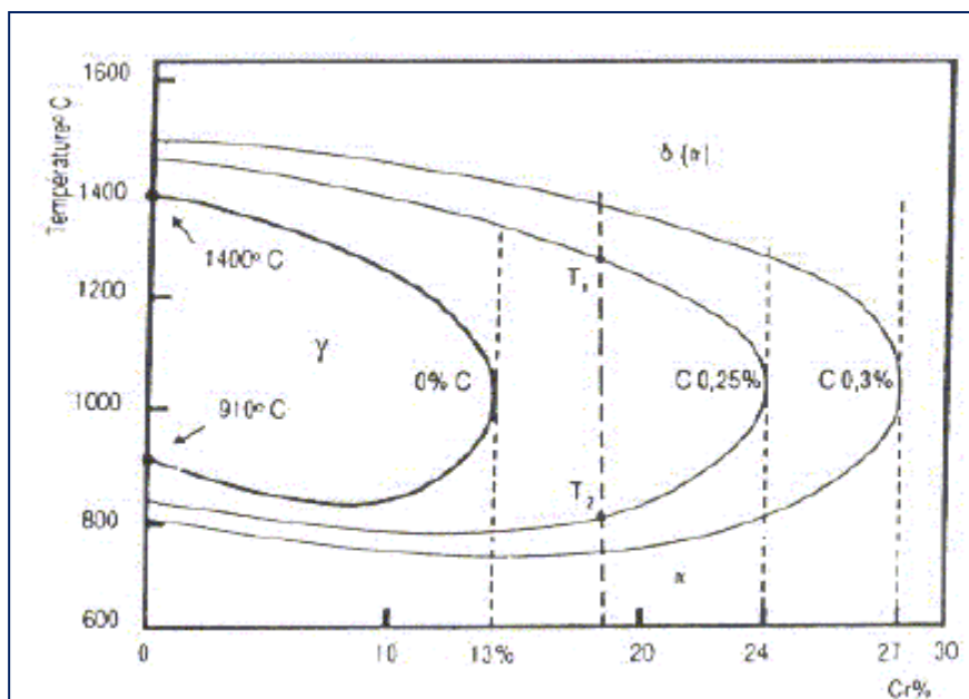
Figure 1.2 : Projection sur le plan température/teneur en chrome des coupes du diagramme Fe-Cr-C pour des teneurs croissantes en carbone [15].
