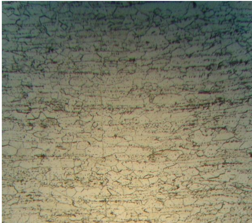
Figure 3.2.a Micrographie d'un échantillon déformé à 15% suivi d'un recuit à 600°C
