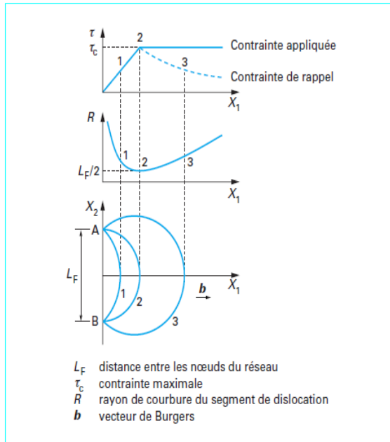
Figure 1.16. : Variation de la contrainte de résistance due à la tension de ligne au cours de la dilatation du segment actif dans le réseau de Frank [31]
