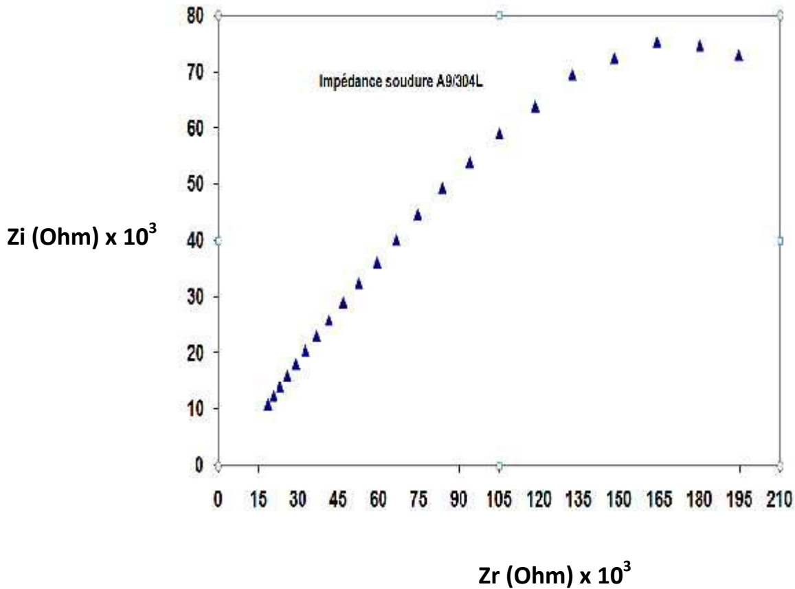
Figure II.17 : Courbe d'impédance de Nyquist, Soudure A9/304L.
