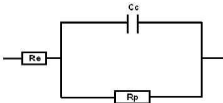
Figure II.12 : Schéma électrique équivalent d'un système avec revêtement poreux sans interface métal / électrolyte. [62]
